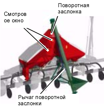
Запорные задвижки
