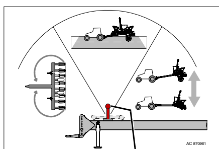
Положение „Транспортировка“
